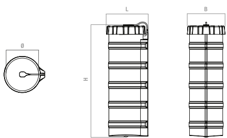
Zeichnung für A500165
