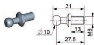
Kugelzapfen - verzinkt
