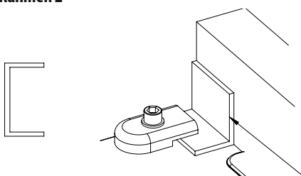
Rahmen 2
