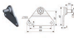
Seitenbeschlag - verzinkt
