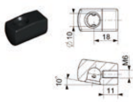
Winkelgelenk (10°) - Kunststoff
