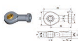
Gelenkkopf - verzinkt
